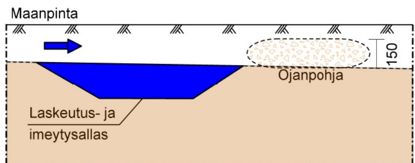
Ojaan rakennetaan pohjakynnyksiä, jotka ohjaavat vettä sivu-uomiin. Kynnyksen etupuolelle kaivetaan laskeutus- ja imeytysallas, johon jää veden mukanaan kuljettamia kiintoaineita ja ravinteita.
