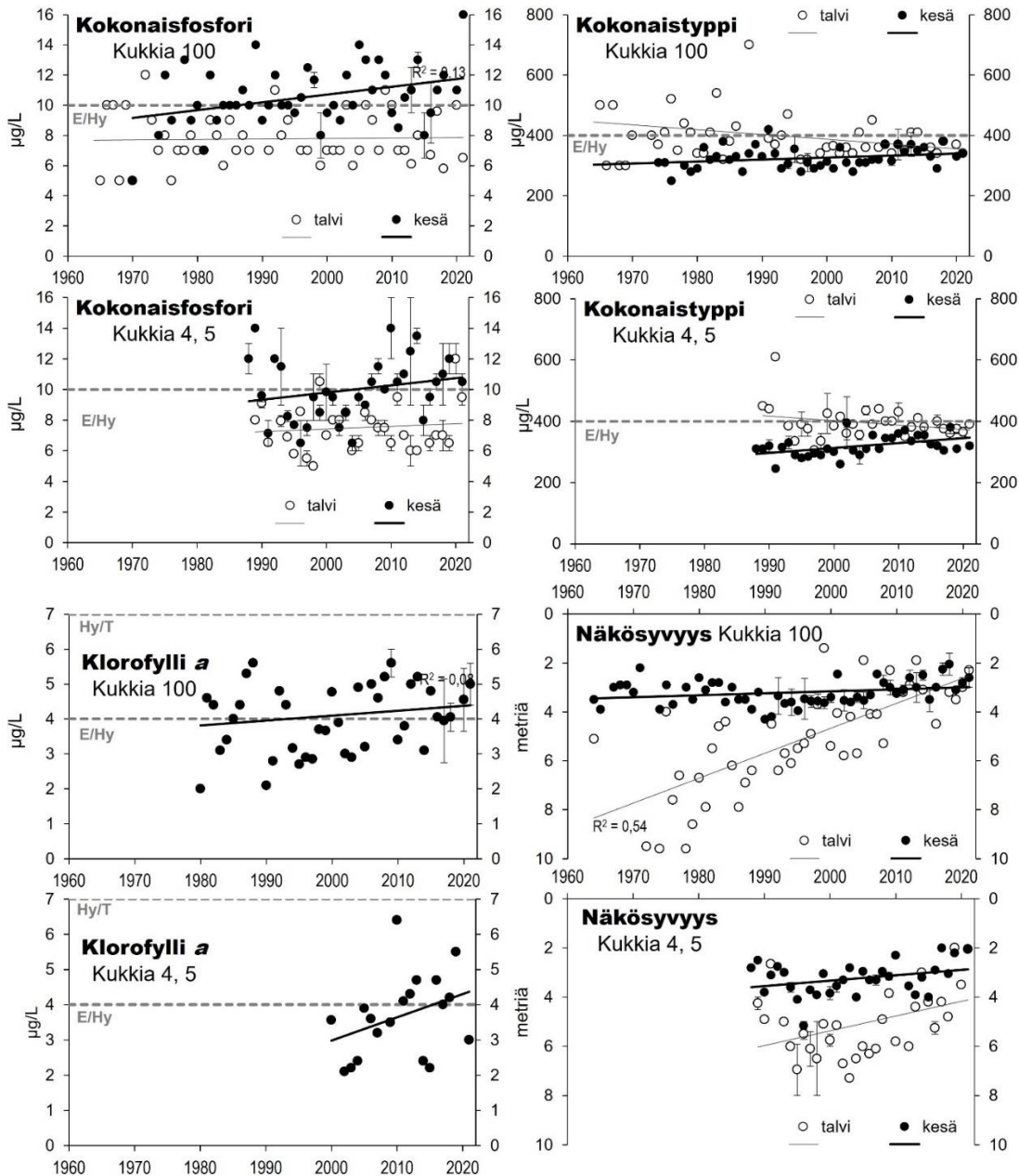
Kuva 15: Kokonaisfosforin ja -tyypin sekä levämäärää ilmentävän klorofylli a -pigmentin pitoisuudet ja näkösyvyys, pintavedessä Kukkien läntisessä järvaltaassa sijaitsevista kolmesta havaintopisteestä ”Kukkia 100”, ”Kukkia 4” ja ”Kukkia 5”, joista jälkimmäisten kahden tulokset on yhdistetty ja laskettu vuosittain keskiarvoiksi ( \pm keskiarvon keskivirheet) talvi- ja kesäkerrostuneisuuskausien lopulla vuosien 1964 ja 2021 välisenä ajanjaksona. Suurten vähähumuksisten järvien ekologisen tilan luokittelun raja-arvot näkyvät katkoviivoina ravinne- ja klorofyllipitoisuuksia esittävässä kuvassa (E = erinomainen, Hy = hyvä).
