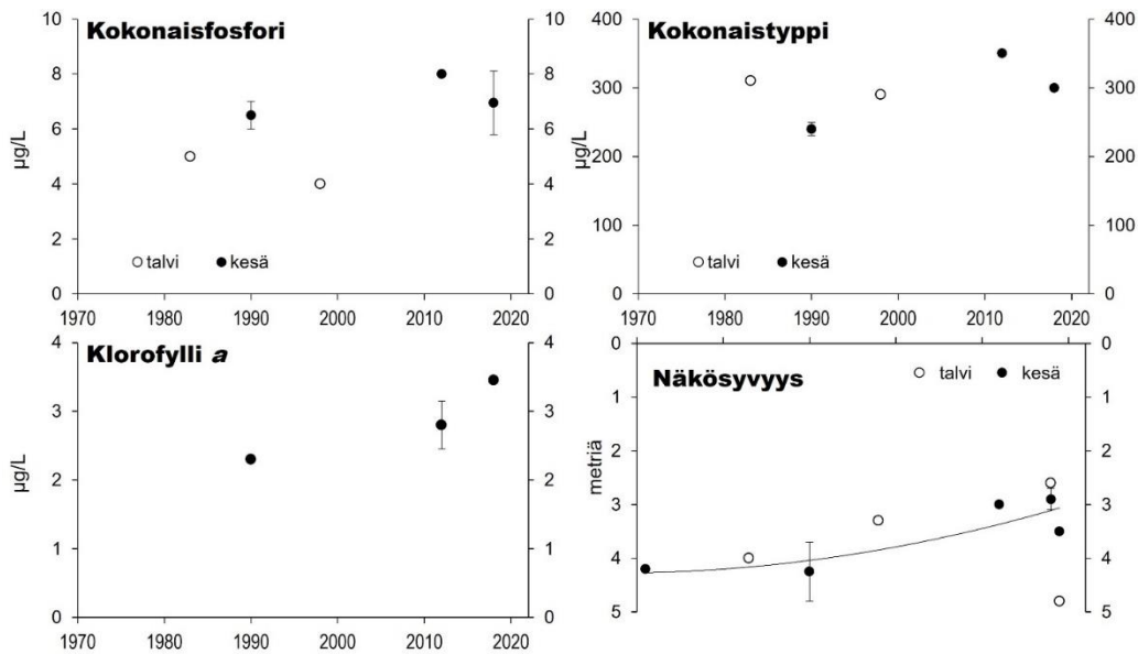
Kuva 11: Kokonaisfosforin ja -typen pitoisuudet sekä levämäärää ilmentävän klorofylli a -pigmentin pitoisuudet ja näkösyvyys pintavedessä keskellä Kyynäröjärveä sijaitsevassa havaintopisteessä talvi- ja kesäkerrostuneisuuskausien lopulla vuosien 1971 ja 2018 välisenä ajanjaksona. Ekologisen tilan luokittelun raja-arvoja ei ole piirretty diagrammeihin, koska Kyynäröjärven kaikki vedenlaatua kuvaavat ominaisuudet osoittavat erinomaista tilaa (eli kaikki mittaustulokset ovat erinomaisen/hyvän raja-arvon alapuolella).
