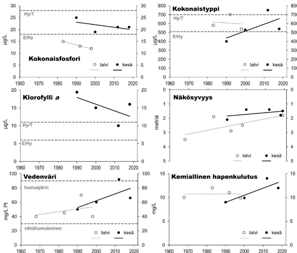
Kuva 9. Kokonaisfosforin ja -tyypin sekä levämäärää ilmentävän klorofylli a -pigmentin pitoisuudet, näkösyvyys ja vedenväri sekä kemiallinen hapenkulutus pintavedessä keskellä Ämmätsänjärveä sijaitsevassa havaintopisteessä talvi-
