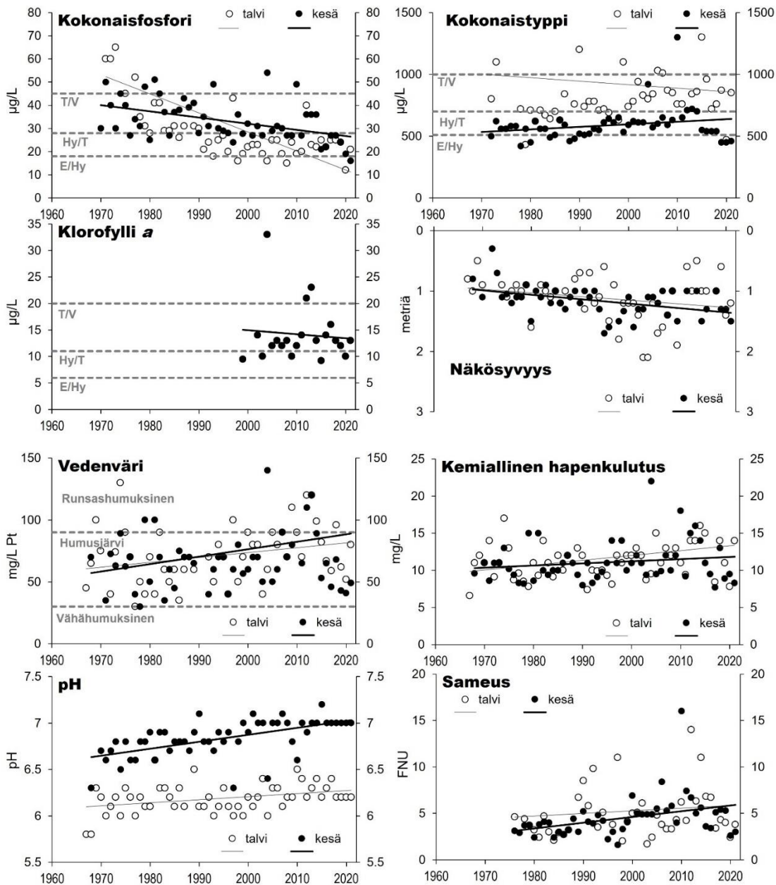
Kuva 13: Kokonaisfosforin ja -tyypin sekä levämäärää ilmentävän klorofylli a -pigmentin pitoisuudet, näkösyyvyys, vedenväri, kemiallinen hapenkulutus, pH ja sameus pintavedessä keskellä Rautajärveä sijaitsevassa havaintopisteessä talvi- ja kesäkerrostuneisuuskausien lopulla vuosien 1967 ja 2021 välisenä ajanjaksona. Pienten humusjärvien ekologisen tilan luokittelun raja-arvot näkyvät katkoviivoina ravinne- ja klorofyllipitoisuuksia esittävässä kuvassa (E = erinomainen, Hy = hyvä, T = tyydyttävä ja V = välttävä).
