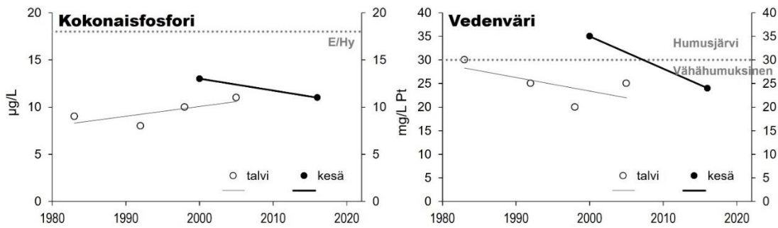
Kuva 20: Kokonaisfosforin pitoisuus ja vedenväri pintavedessä Vekunassa talvi- ja kesäkerrostuneisuuskausien lopulla vuosien 1983 ja 2016 välisenä ajanjaksona. Pienten vähähumuksisten järvien ekologisen tilan luokittelun erinomaisen/hyvän raja-arvo näkyy katkoviivana fosforipitoisuuksia esittävässä diagrammissa. Vähähumuksisen järven ja humusjärven raja-arvo vedenvärin perusteella arvioituna näkyy katkoviivana vedenväriä esittävässä diagrammissa. (Vekunan pintaveden kokonaistyyppipitoisuus on n. 200 µg/l)
