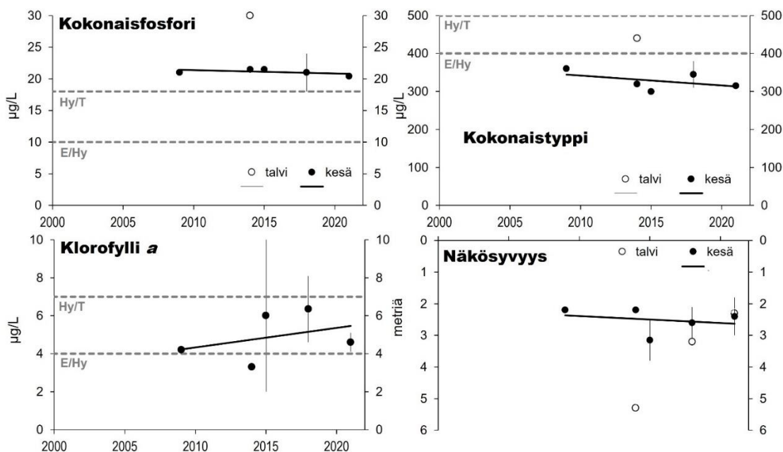
Kuva 37: Pintaveden (1 m) kokonaisfosforin ja -tyypin sekä levämäärää ilmentävän klorofylli a -pigmentin pitoisuuksien ja näkösyvyyden keskiarvo (±keskiarvon keskivirheet) Roineen Tossanselän keskellä olevasta ”Roine Tossanselkä” -
