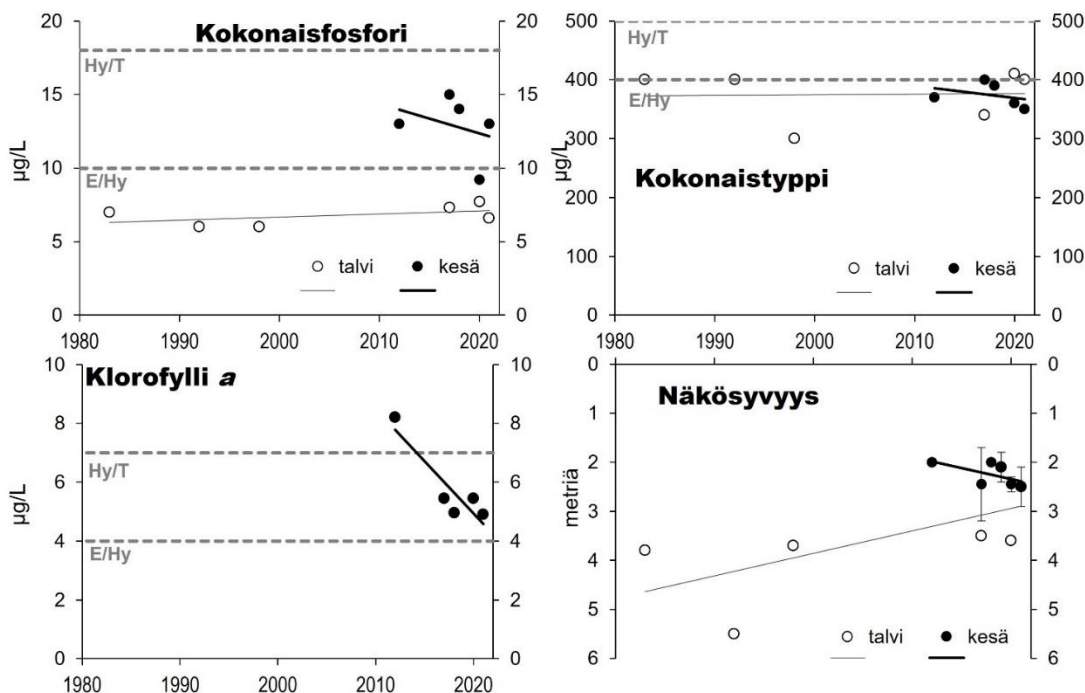
Kuva 18: Kokonaisfosforin ja -tyypin sekä levämäärää ilmentävän klorofylli a -pigmentin pitoisuudet ja näkösyvyys Vihajärvessä talvi- ja kesäkerrostuneisuuskausien lopulla vuosien 1983 ja 2021 välisenä ajanjaksona. Pienten
