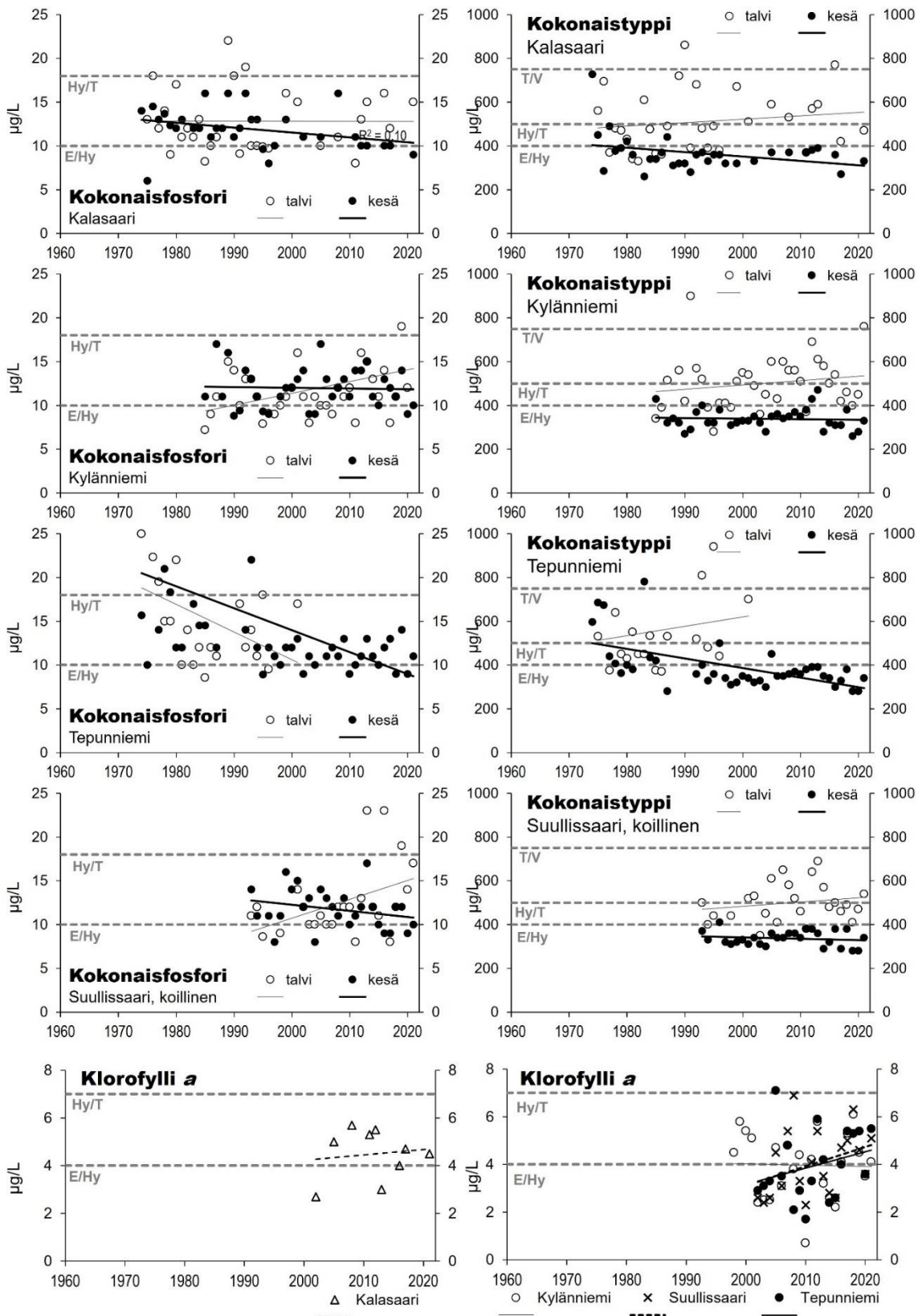
Kuva 30: Kokonaisfosforin ja -tyypin sekä levämäärää ilmentävän klorofylli a -pigmentin pitoisuudet pintavedessä Pälkäneveden Jouttesselän neljässä havaintopisteessä talvi- ja kesäkerrostuneisuuskausien lopulla vuosien 1962 ja 2021 välisenä ajanjaksona. Pienten ja keskikokoisten vähähumuksisten järvien ekologisten tilan luokittelun raja-arvot näkyvät katkoviivoina ravinne- ja klorofyllipitoisuuksia esittävissä kuvissa (E = erinomainen, Hy = hyvä, T = tyydyttävä ja V = välttävä).
