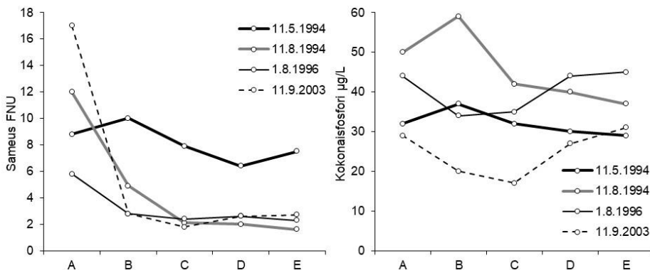
Kuva 26: Sameus ja kokonaisfosfori Pitkälähdellä.
