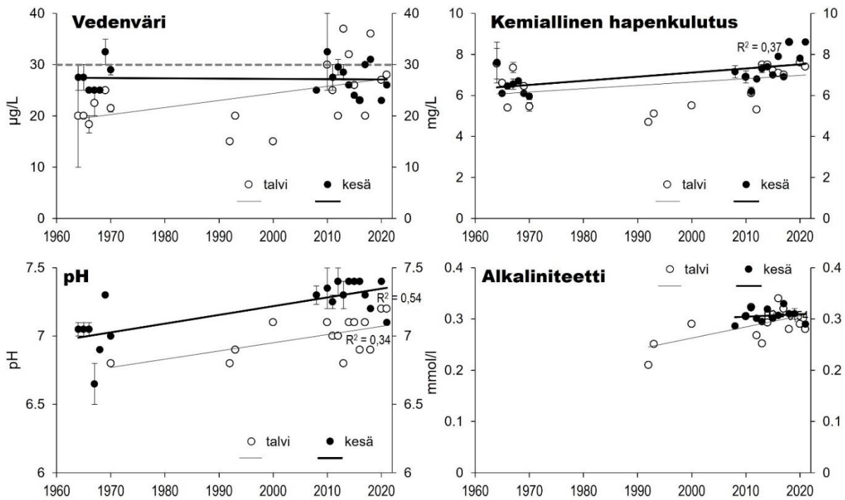
Kuva 35: Pintaveden (1 m) kokonaisfosforin ja -typen sekä levämäärää ilmentävän klorofylli a -pigmentin pitoisuuksien, näkösyvyyden, veden värin, kemiallisen hapenkulutuksen, pH:n ja alkaliniteetin keskiarvo ( \pm keskiarvon keskiarvo) Pinteleen kahdessa havaintopisteessä talvi- ja kesäkerrostuneisuuskausien lopulla vuosien 1964 ja 2021 välisenä ajanjaksona. Pienten ja keskikokoisten vähähumuksisten järvien ekologisten tilan luokittelun raja-arvot näkyvät katkoviivoina ravinne- ja klorofyllipitoisuuksia esittävässä kuvissa (E = erinomainen, Hy = hyvä, T = tyydyttävä).
