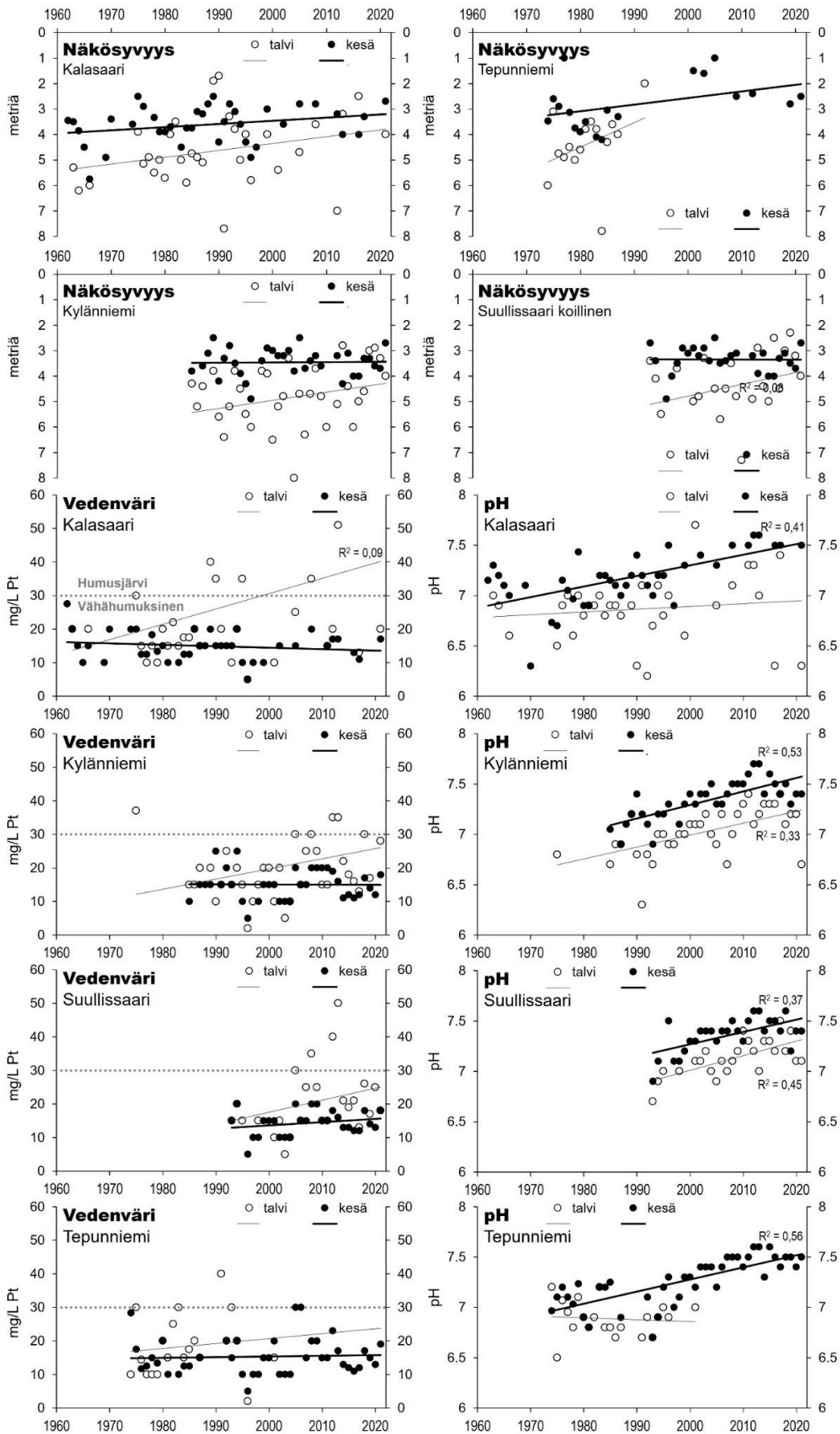
Kuva 31: Näkösyvyys, veden väri ja pH pintavedessä Pälkäneveden Jouttesselän neljässä havaintopisteessä talvi- ja kesäkerrostuneisuuskausien lopulla vuosien 1962 ja 2021 välisenä ajanjaksona.
