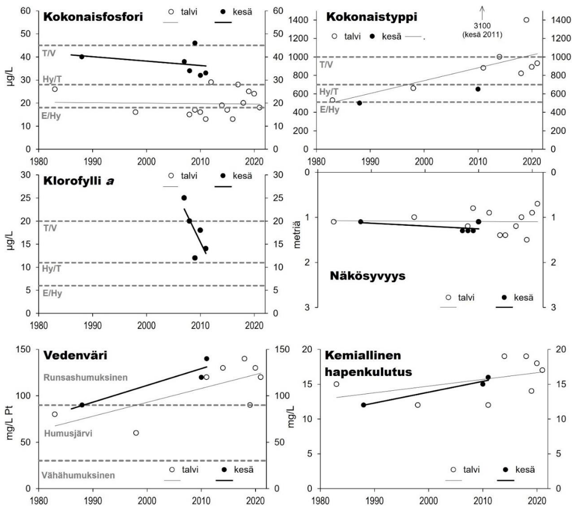
Kuva 28: Kokonaisfosforin ja -tyypin pitoisuus sekä levämäärää ilmentävän klorofylli a -pigmentin pitoisuudet, näkösyvyys, vedenväri ja kemiallinen hapenkulutus pintavedessä Sappeenjärven Taivallahdessa sijaitsevassa havaintopisteessä talvi- ja kesäkerrostuneisuuskausien lopulla vuosien 1983 ja 2021 välisenä ajanjaksona. Pienten humusjärvien ekologisten tilan luokittelun raja-arvot näkyvät katkoviivoina ravinne- ja klorofyllipitoisuuksia esittävässä kuvissa (E = erinomainen, Hy = hyvä, T = tyydyttävä ja V = välttävä). Vedenväriä osoittavassa diagrammissa on lisäksi raja-arvot, joilla järvi luokitellaan humuspitoisuuden suhteen
