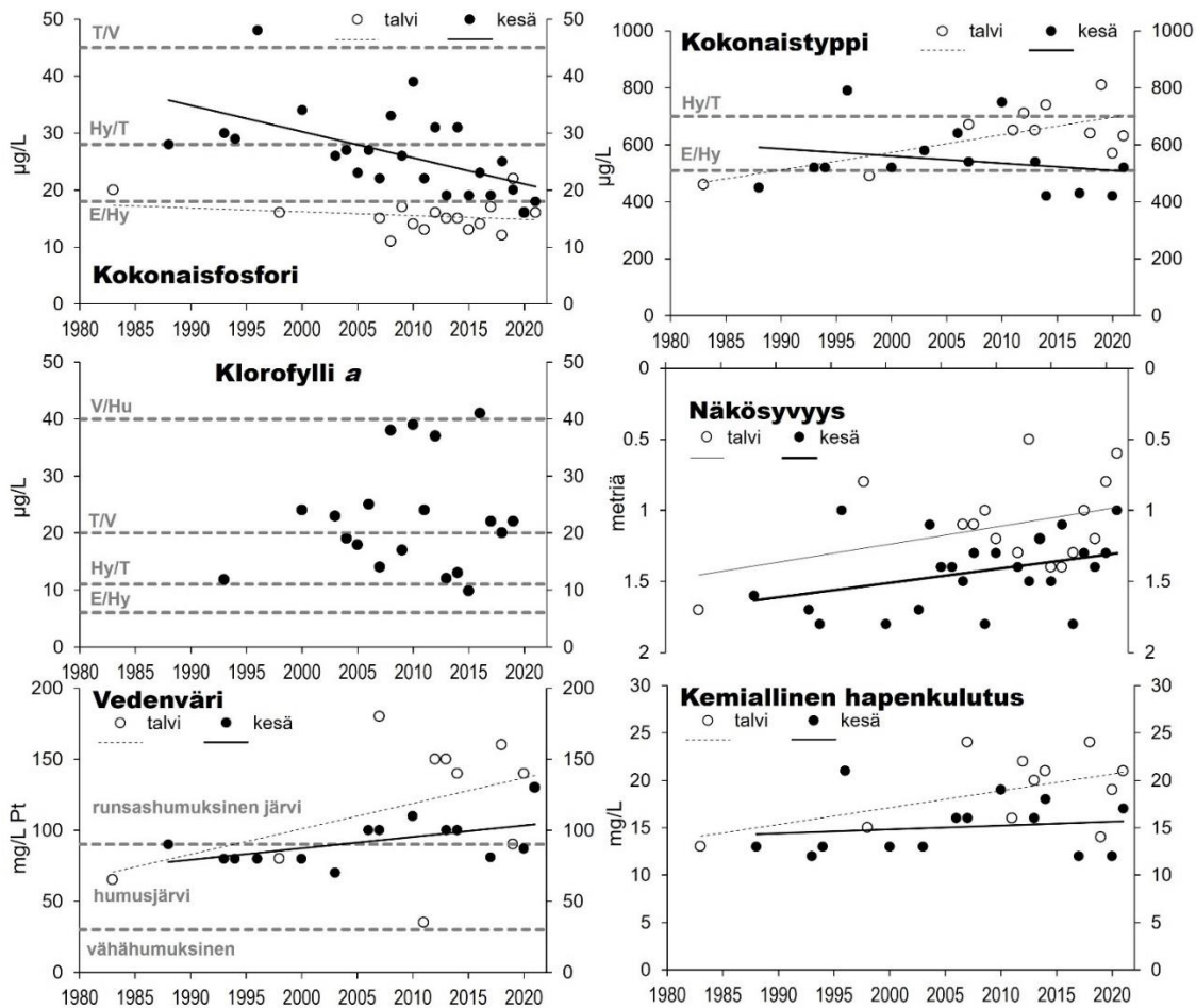
Kuva 24: Kokonaisfosforin ja -tyypin sekä levämäärää ilmentävän klorofylli a -pigmentin pitoisuudet, näkösyvyys, vedenväri ja kemiallinen hapenkulutus pintavedessä keskellä Iso Arajärveä sijaitsevassa havaintopisteessä talvi- ja kesäkerrostuneisuuskausien lopulla vuosien 1983 ja 2021 välisenä ajanjaksona. Pienten humusjärvien ekologisen tilan luokittelun raja-arvot näkyvät katkoviivoina ravinne- ja klorofyllipitoisuuksia esittävässä kuvissa (E = erinomainen, Hy = hyvä, T = tyydyttävä, V = välttävä, Hu = huono). Vedenväriä osoittavassa diagrammissa on lisäksi raja-arvot, joilla järvi luokitellaan humuspitoisuuden suhteen.
